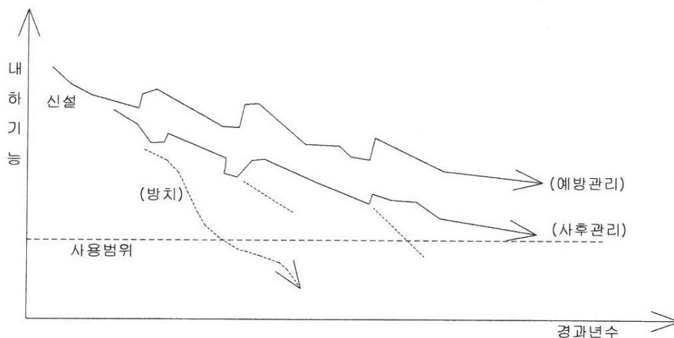
[그림1] 시간경과에 따른 건축물의 내하기능 저하
